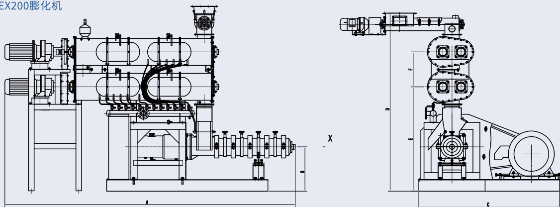
SREX200膨化机
