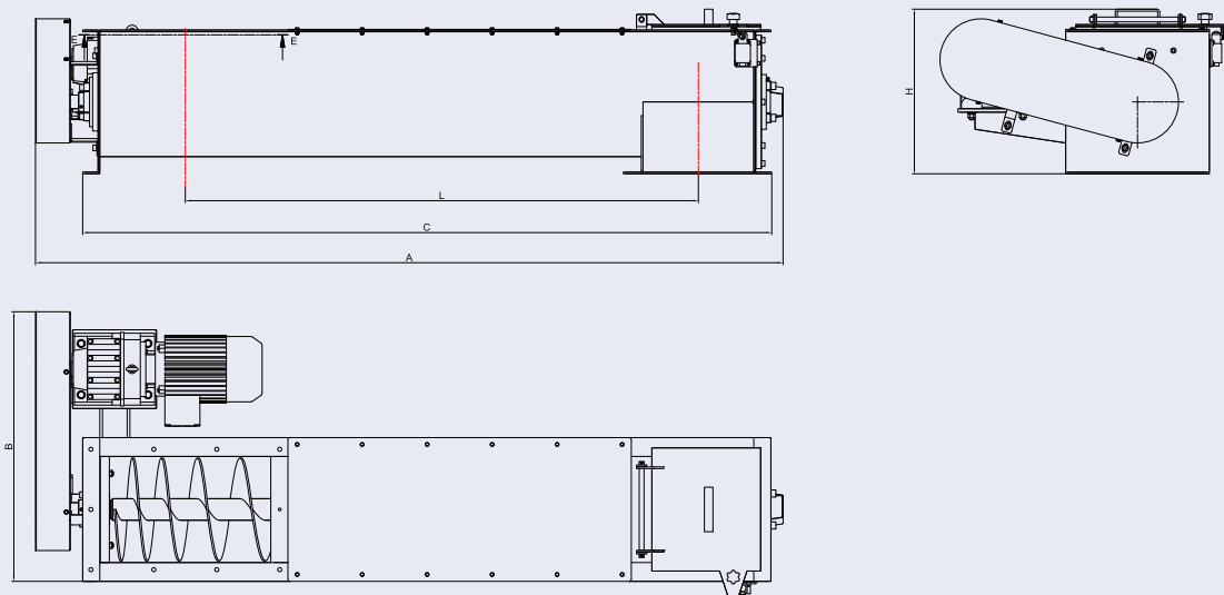
SFB300 螺旋喂料器
