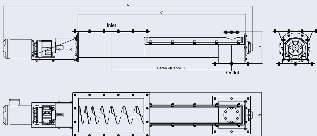
SF系列螺旋喂料器
