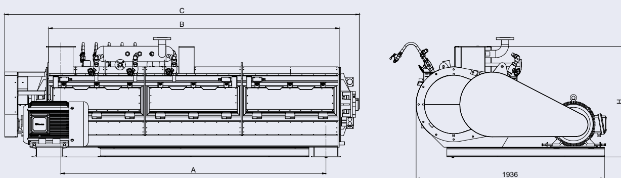
SDDC调质器
